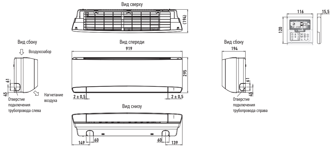
CS-Z25YKEA / CS-Z35YKEA
