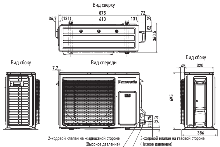
CU-Z50YKEA / CU-Z71YKEA
